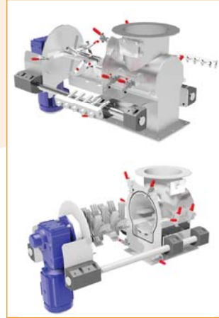
Links boven PPB-300R-1 Links onder PMBR-300-1 Rechtsboven de brekeras met ronde pennen daaronder is de veegbreker PVB-300-1
