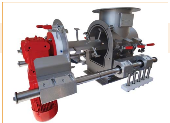
Precision PVB-300R-1 de veegbreker is een uitvoering waar de kleinere harde agglomeraat deeltjes door een veegbeweging door het zeefdek worden gedrukt. Een toepassing die veel bij kristalsuiker agglomeraten is gebruikt.
